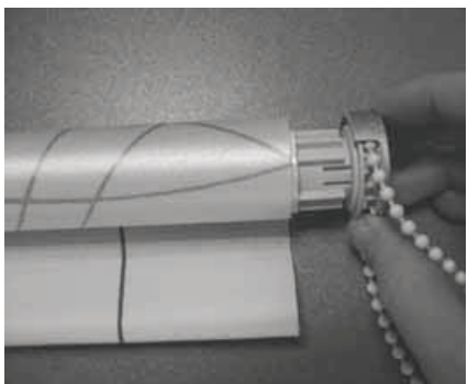
Kædetrækket monteres igen i rullegardinsrøret
