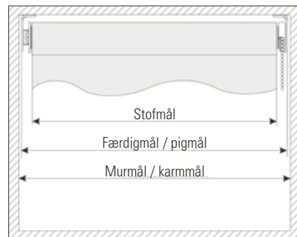
Målangivelser for Faber rullegardiner med kædetræk
