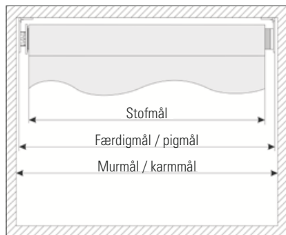
Målangivelser for Faber rullegardiner med fjeder
